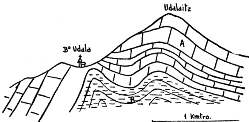
CORTE GEOLOGICO DE UDALAITZ: «A», Calizas Urganianas, «B», Arcillas negras Wealdienes.
