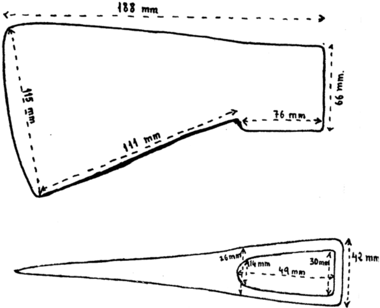
HACHA DE HIERRO: Difiere en algunas de sus características
