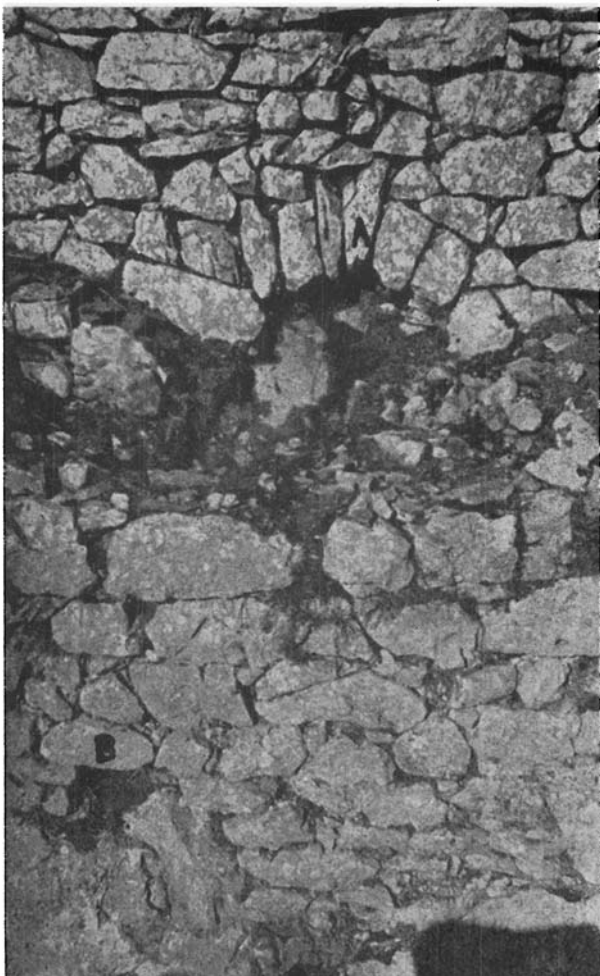
Foto 7. — Al realizar una cata, apareció una hilera de tejas invertidas, entre A y B, en forma de conducción de aguas
